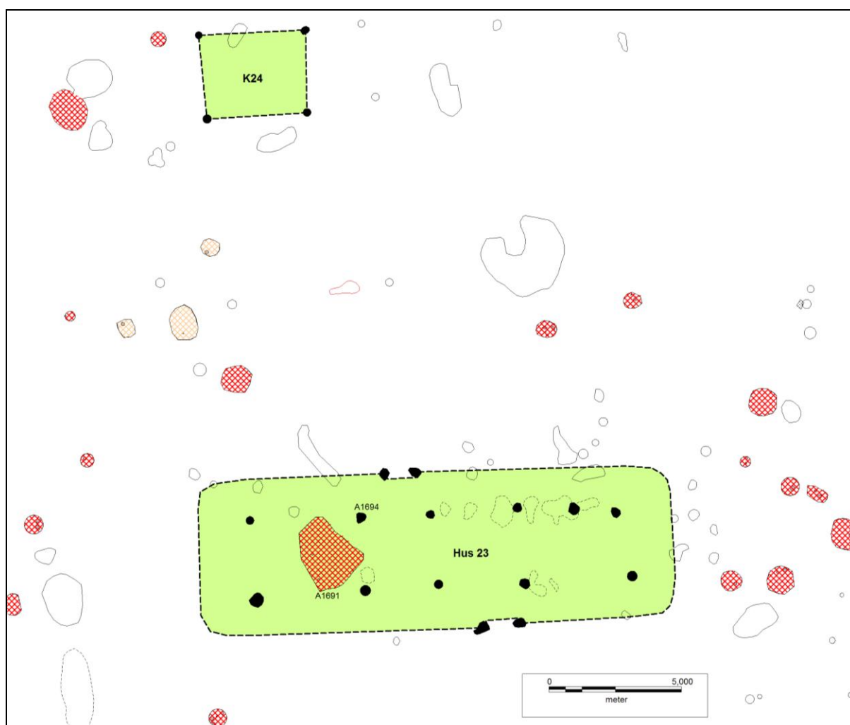
Plan over gård fra yngre bronzealder bestående af Hus 23 og den mindre bygning K24. I tagstolpehul A1694 blev der fundet lerkarskår. De sortfarvede anlæg er stolpehuller til husene, mens de anlæg der er skrårskraveret røde og orange er ild-/kogegruber.
