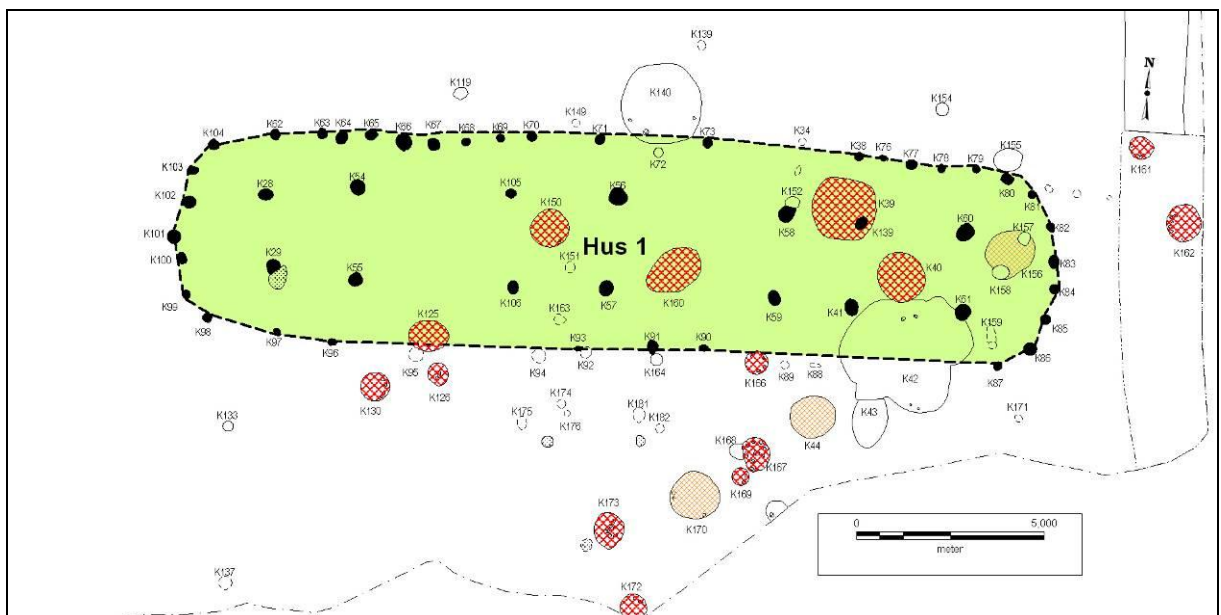
Plan over Hus 1. De sortfarvede anlæg er stolpehuller til huset, mens de anlæg, der er skråskraveret røde eller orange er ældre ild-/kogegruber.
