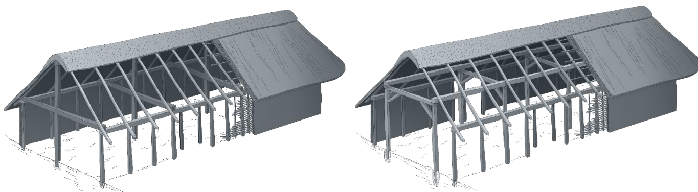
Figur 6. Rekonstruktionstegning af et midtsulehus med en række tagstolper i midten af huset, og et treskibet langhus med sætvis tagbærende stolper. I forgrunden er nedgravningerne til stolperne markeret, og det er disse vi kan genfinde i dag. Illustration: Jeanette Nørgaard, © Viborg Museum.
