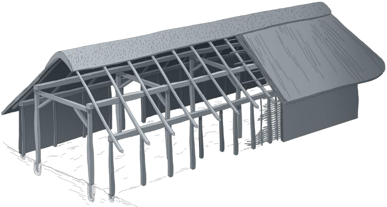
Figur 3. Rekonstruktionstegning af et treskibet langhus med sætvis tagbærende stolper. Illustration: Jeanette Nørgaard, © Viborg Museum.
